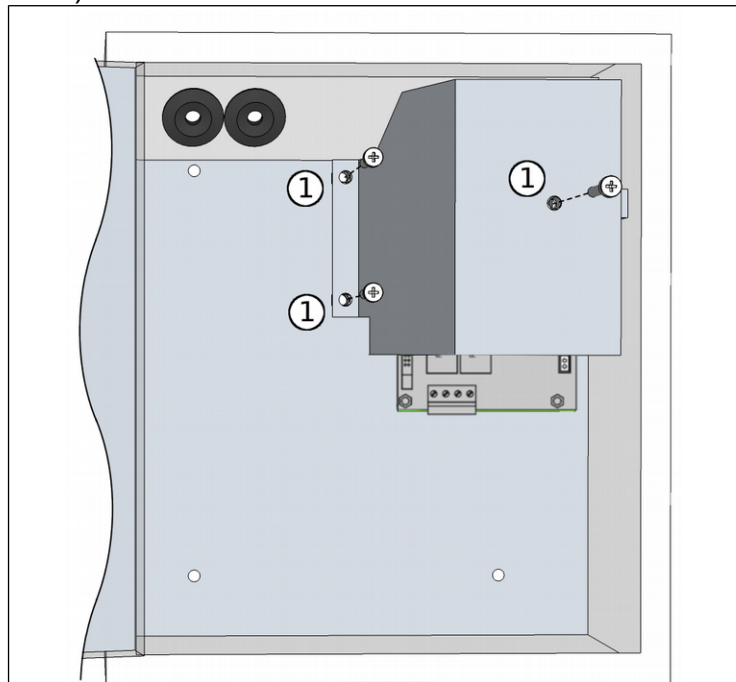
1) Viti di fissaggio della lamiera di protezione
